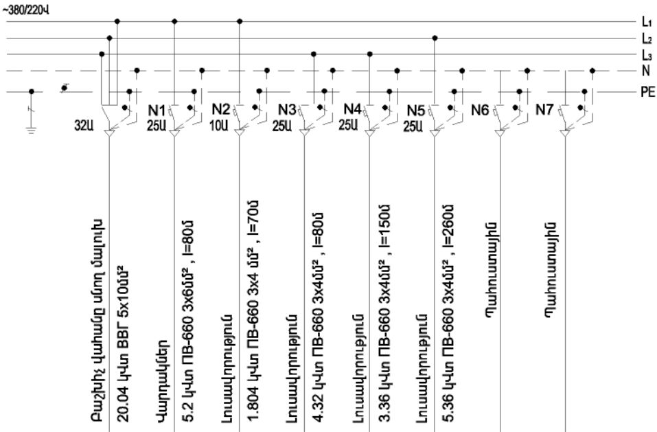
N1 բաշխիչ վահանի սխեմա
