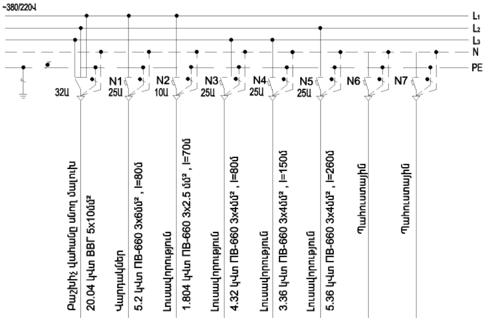
N2 բաշխիչ վահանի սխեմա
