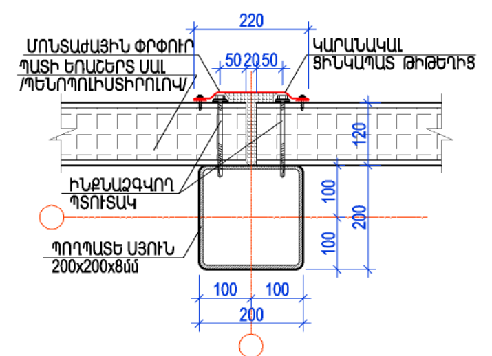
ՀԱՆԳՈՒՅՑ բ
