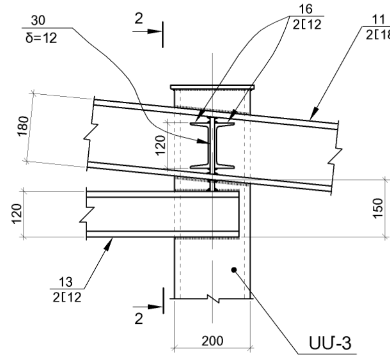
ՀԱՆԳՈՒՅՑ «6» (M 1:10)
