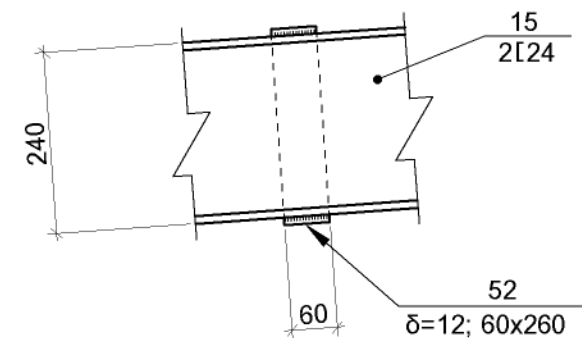
ՀԱՆԳՈՒՅՑ «13» (M 1:10)
