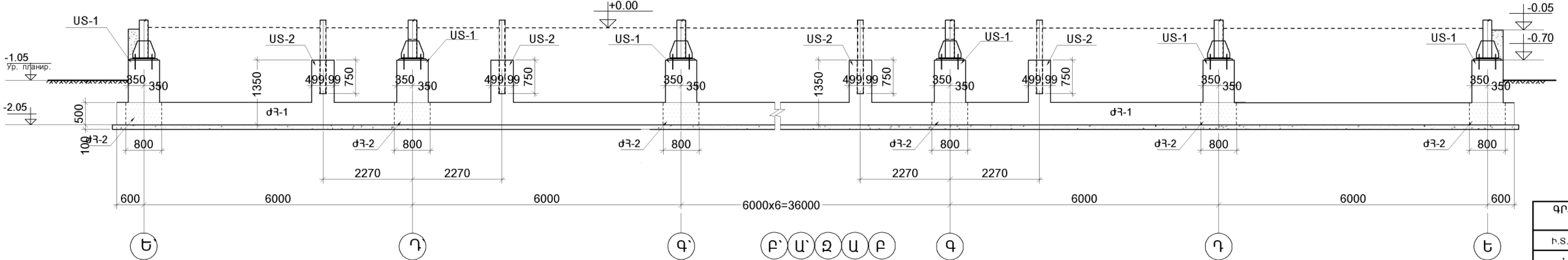
ՓՈՎԱԾՔ "2" ԱՌԱՆՑՔՈՎ
