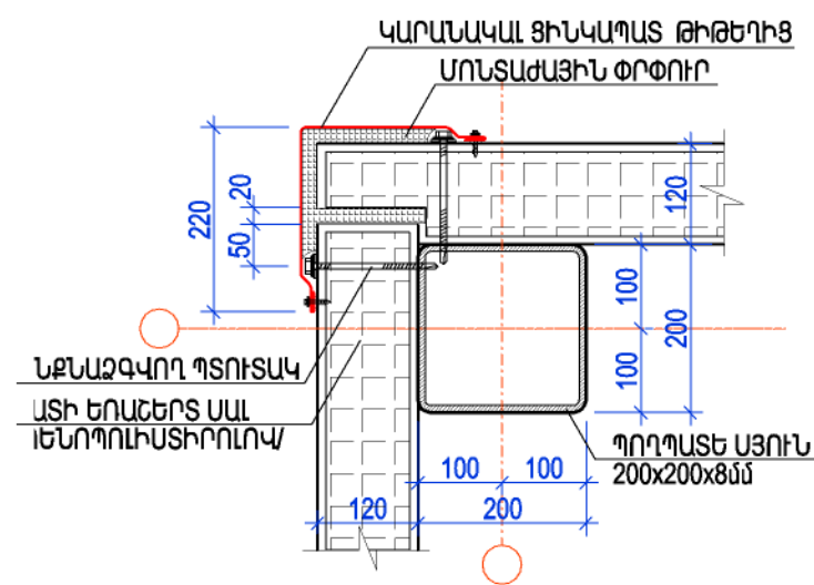
ՀԱՆԳՈՒՅՑ ա
