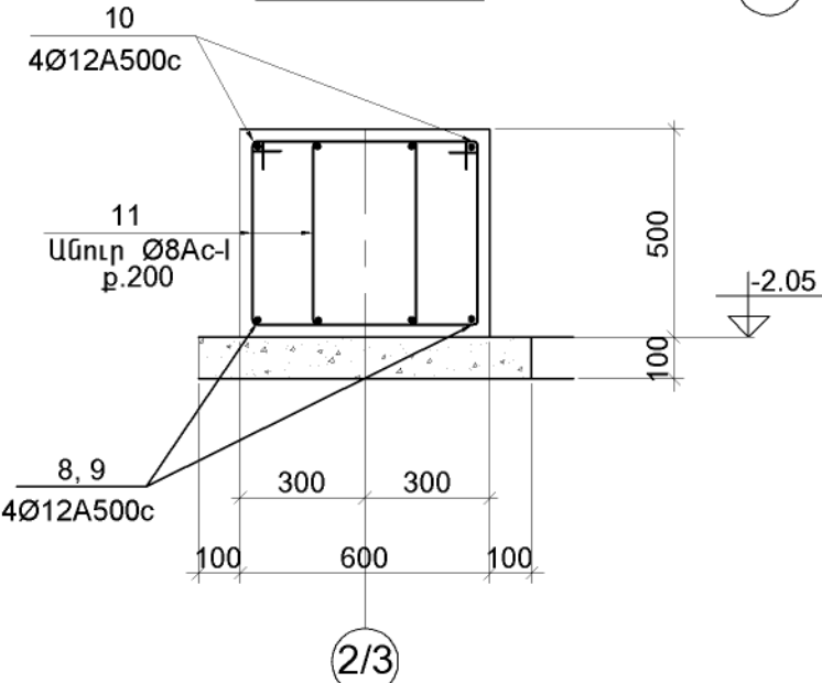
2 - 2 (M1:20)
