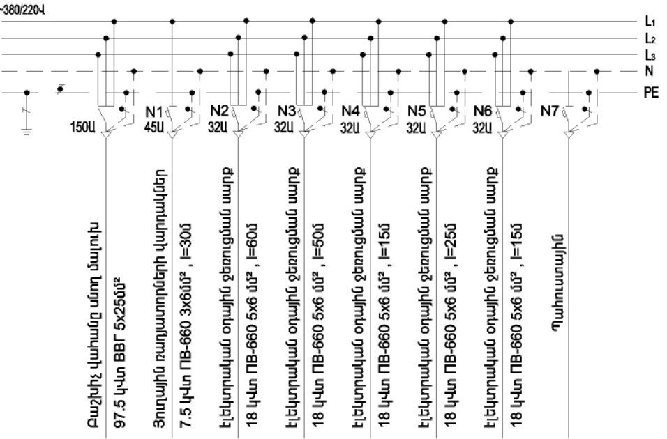
N4 բաշխիչ վահանի սխեմա
