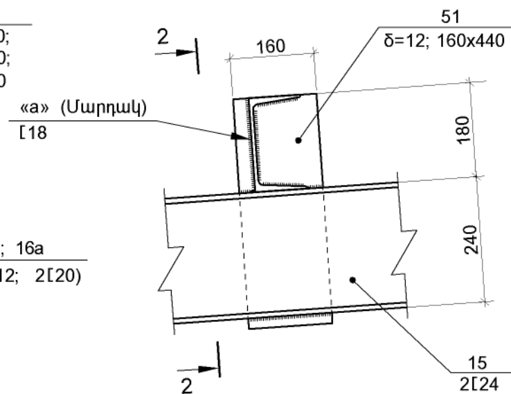
ՀԱՆԳՈՒՅՑ «13» (M 1:10)
