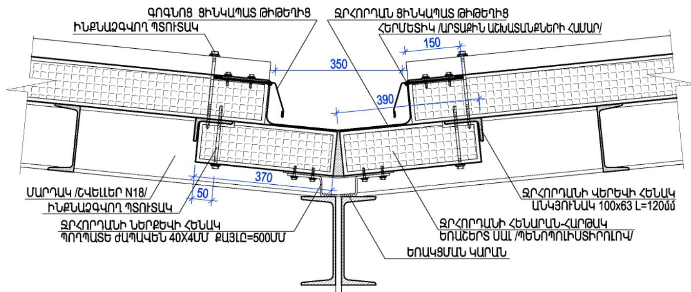
ՀԱՏՈՒՅԹ 1 - 1
