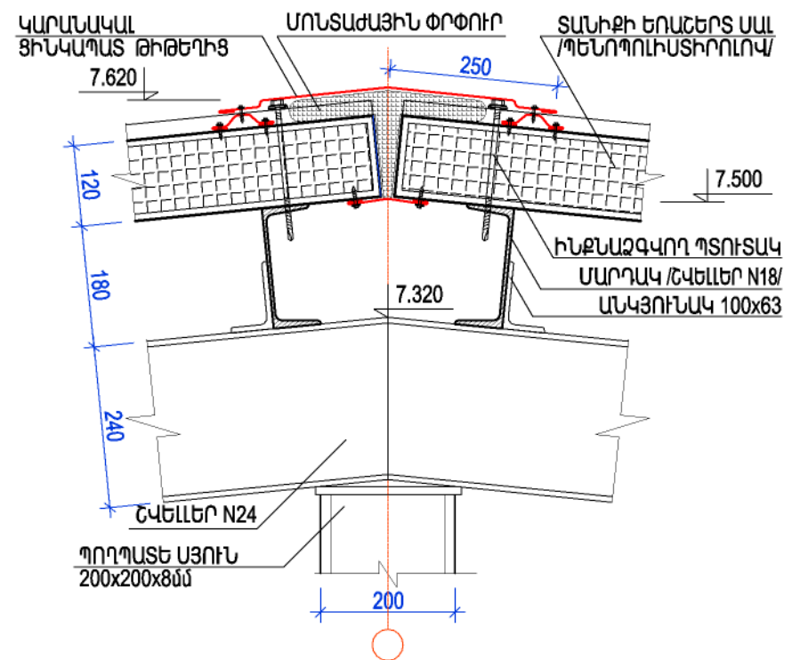
ՀԱՆԳՈՒՅՑ թ
