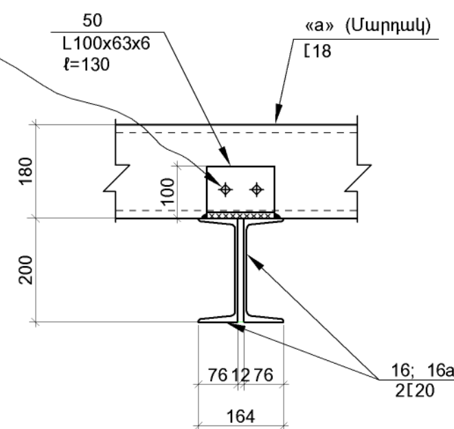
1 - 1
