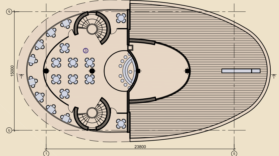
Երկրորդ հարկի հատակագիծ
