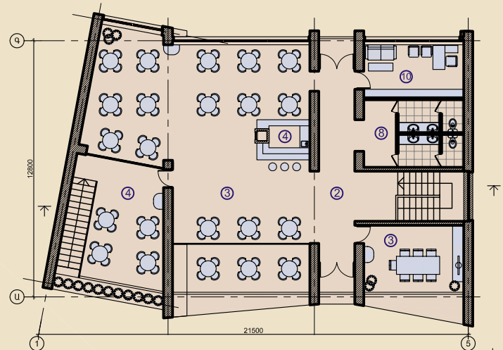
Երկրորդ հարկի հատակագիծ
