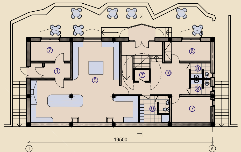
Հատակագիծ -3.00 միշուն
