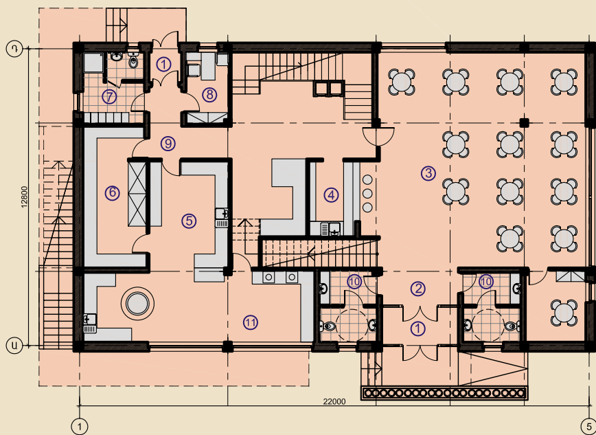
Առաջին հարկի հատակագիծ
