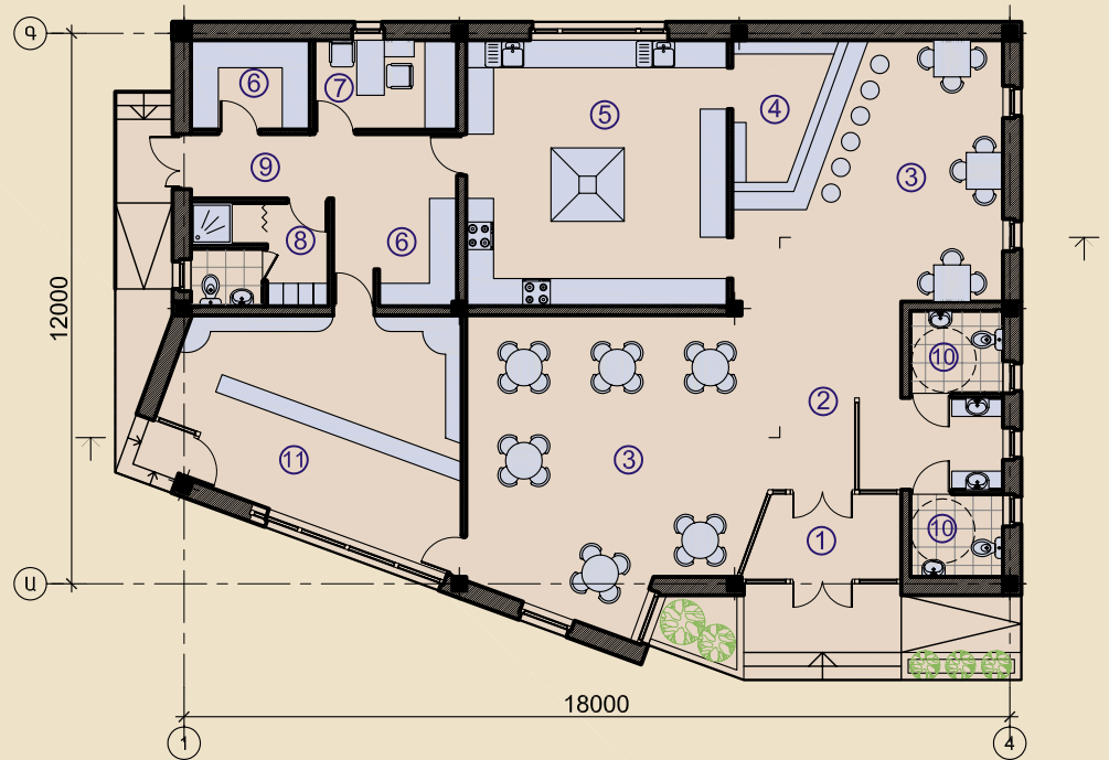
Հատակագիծ
