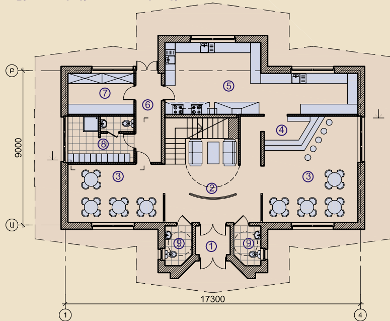
Առաջին հարկի հատակագիծ
