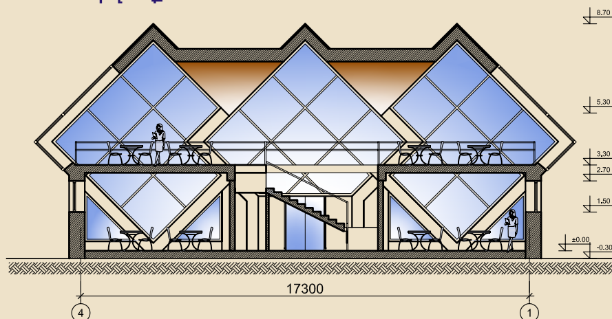
Կտրվածք
