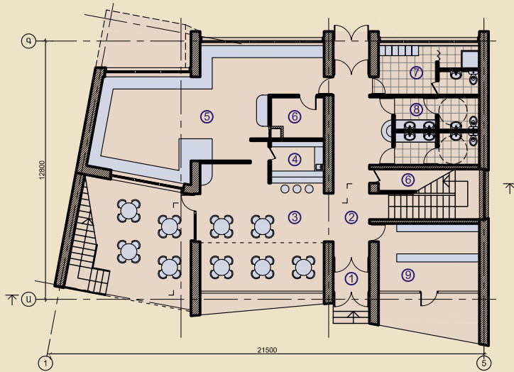
Առաջին հարկի հատակագիծ
