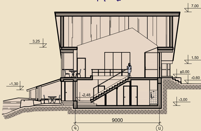
Կտրվածք
