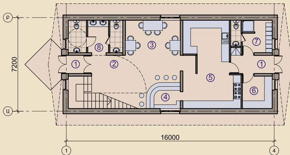
Առաջին հարկի հատակագիծ
