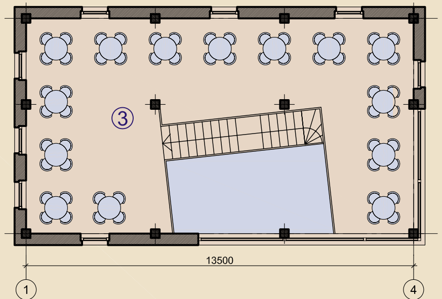
Երկրորդ հարկի հատակագիծ
