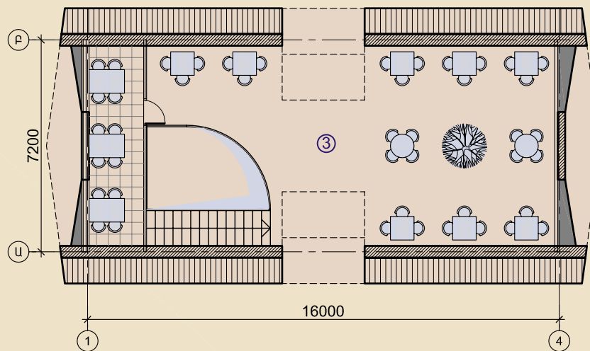
Երկրորդ հարկի հատակագիծ
